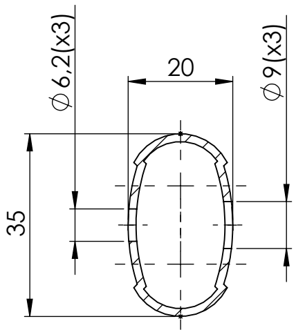
SEZIONE A-A SCALA 1 : 1
