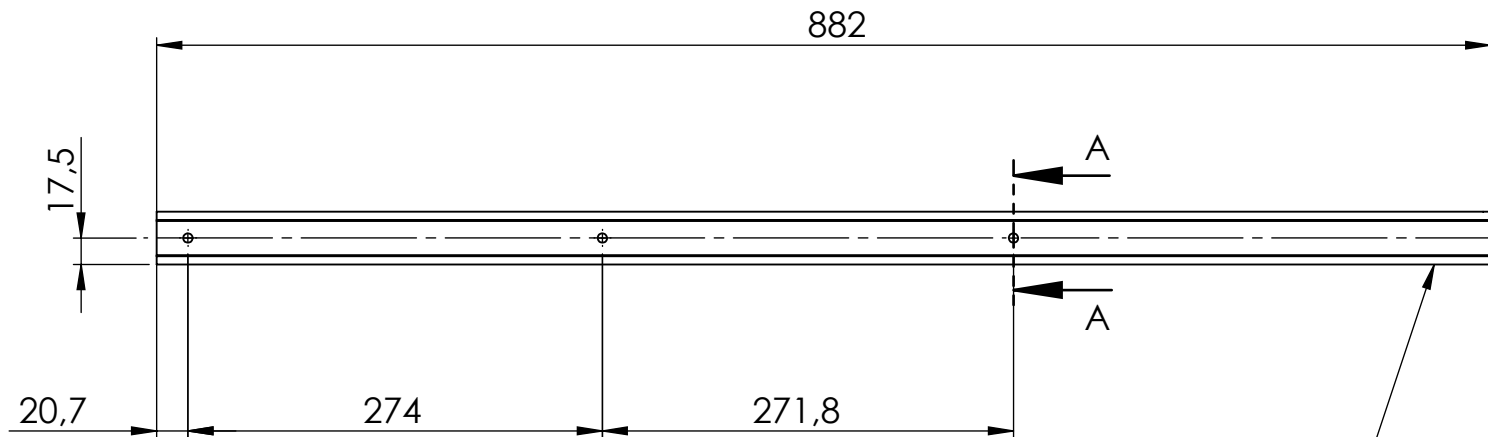
PROFILO COD. -10276
