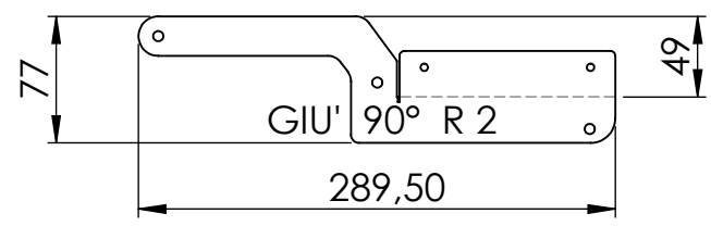
MODELLO DI LAMIERA PIATTO (1:5)
