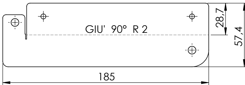
MODELLO DI LAMIERA PIATTO (1:2)
