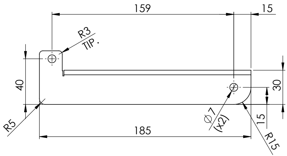
MODELLO DI LAMIERA PIATTO (1:2)
